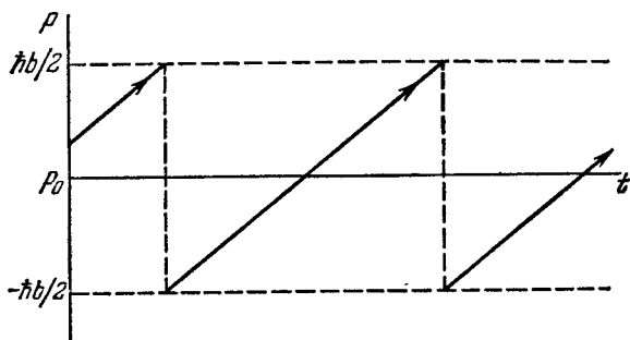
Рис. 4.7. Периодическое движение носителя заряда в зоне Бриллюэна во внешнем электрическом поле (одномерный случай). Сплошные линии изображают траекторию носителя в пространстве квазиимпульсов.
