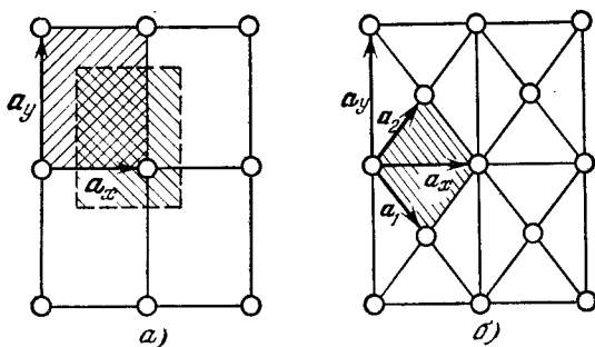
Рис. 2.1. Двумерная прямоугольная решетка: а) простая; б) центрированная. \mathbf{a}_1 , \mathbf{a}_2 — основные векторы решетки Браве.
