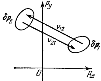
Рис. 7.1. Прямые и обратные электронные переходы.
