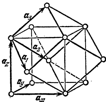
Рис. 2.2. Прямоугольная элементарная ячейка объемноцентрированной кубической решетки (основные векторы \mathbf{a}_x , \mathbf{a}_y , \mathbf{a}_z ) и ромбоэдрическая ячейка решетки Браве (основные векторы \mathbf{a}_1 , \mathbf{a}_2 , \mathbf{a}_3 ).
