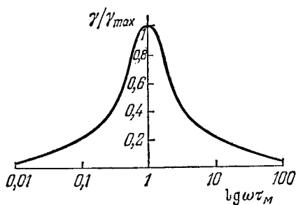
Рис. 15.2. Зависимость электронного коэффициента поглощения звука от \omega\tau_M без внешнего поля.
